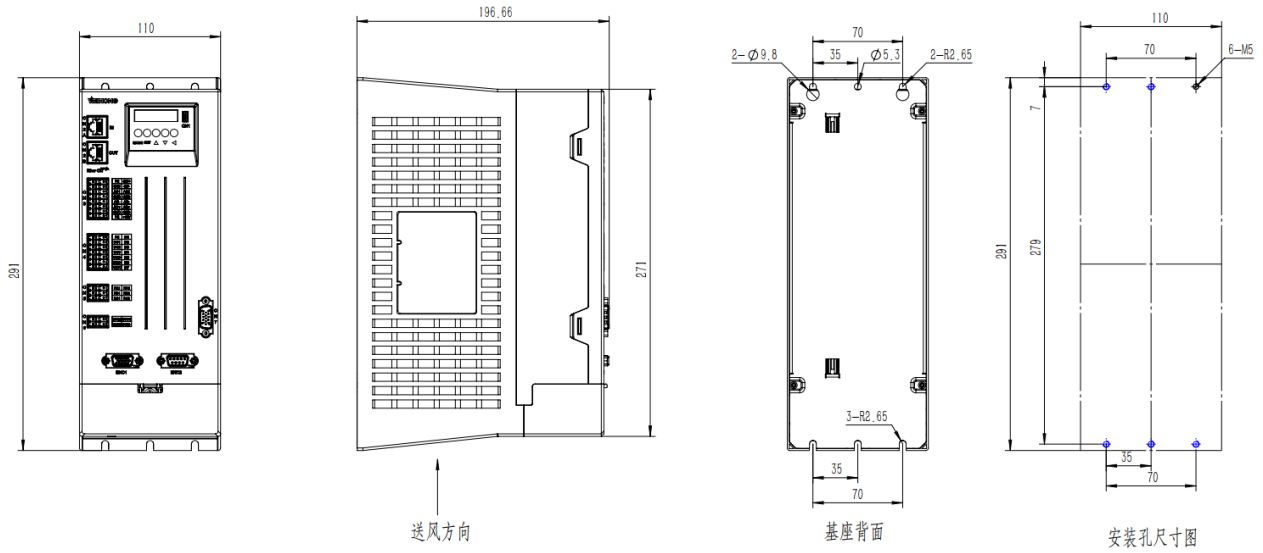
图 2-1 安装尺寸图
