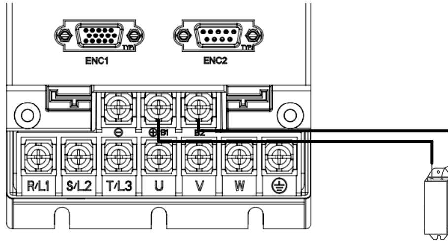
图 3-2 外置再生制动电阻连接示意图
