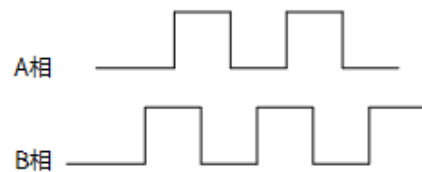
正方向动作
