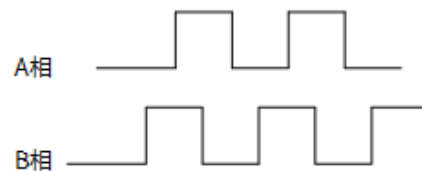
负方向动作
