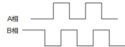
负方向动作
