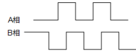
正方向动作
