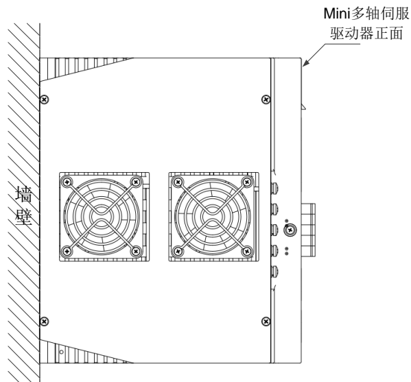
图 2-2 安装方向
