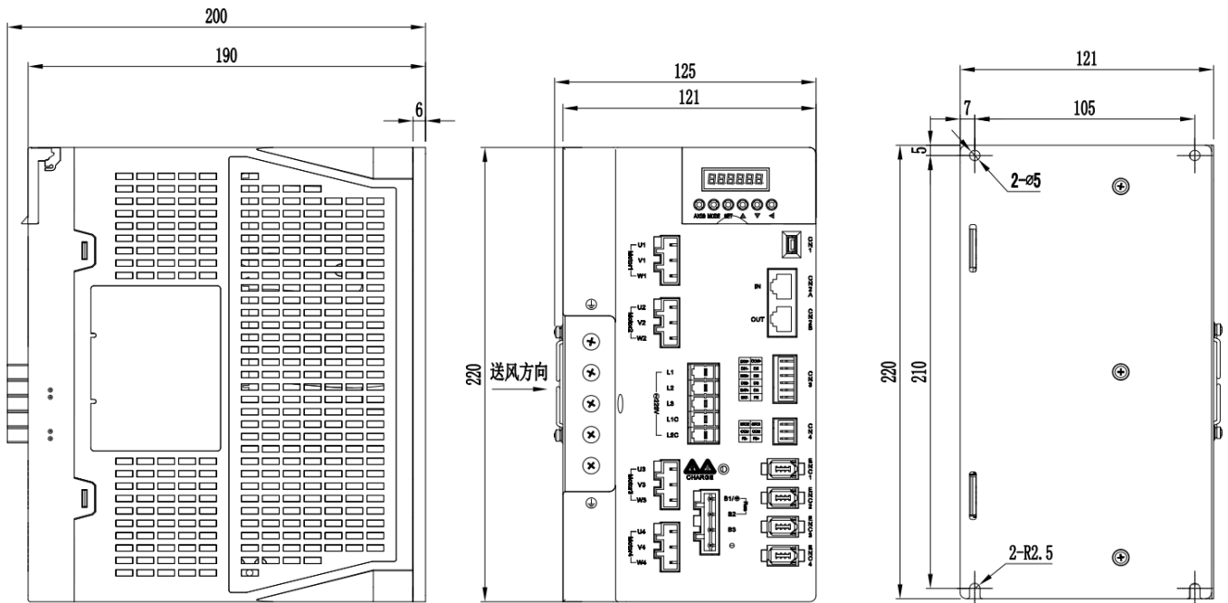
图 2-1 Mini 多轴伺服驱动器安装尺寸图
