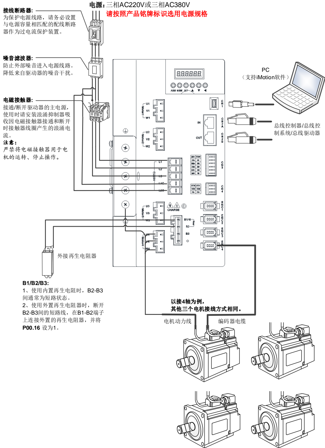
图 1-2 Mini 多轴伺服驱动器与外围设备连接图
